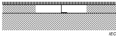
Figure 102b) – SG/SCP pour montage encastré dans le sol – Installé encastré affleurant le niveau le plus élevé du sol
