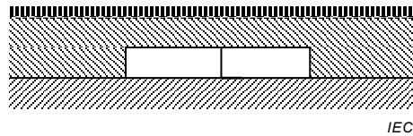
Figure 102a) – SCP pour montage sous le sol – Noyé dans le sol
