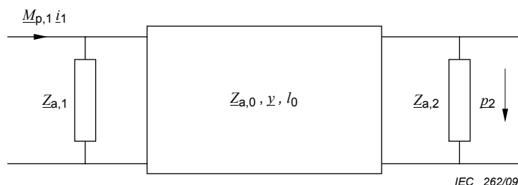
Figure 3 – Circuit équivalent pour évaluer Z'_{a,12} quand on suppose une transmission en ondes planes dans le coupleur
