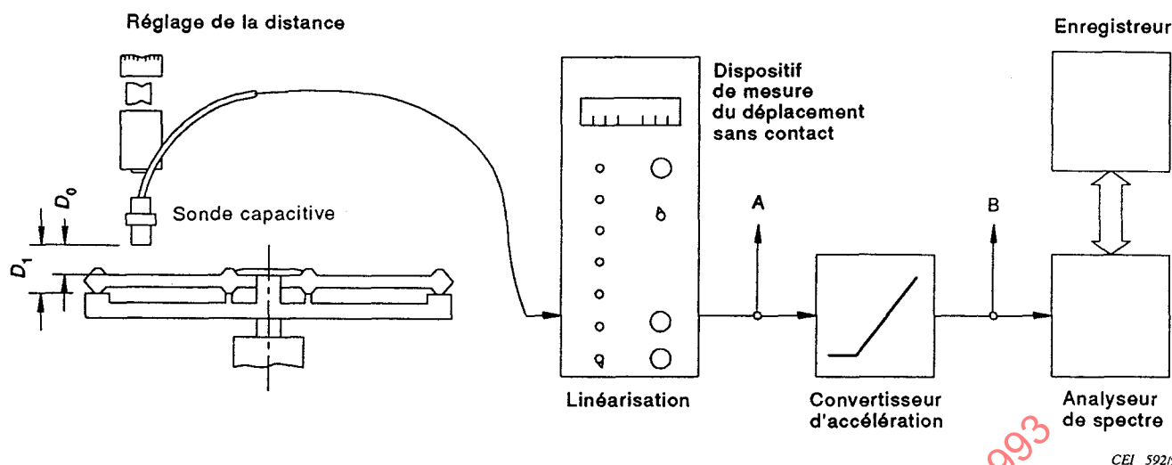
Figure E.1 – Schéma synoptique du dispositif de mesure
