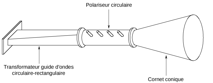
Figure A.1 – Antenne de référence à polarisation circulaire
