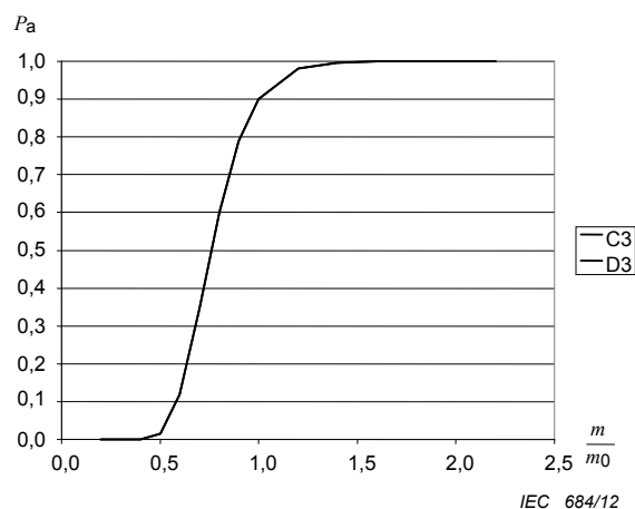
Figure D.12 – Caractéristique d'exploitation P_a
