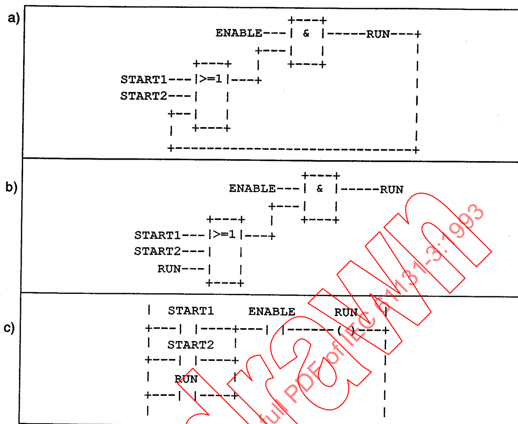
Figure 23 — Exemple de chemin d'asservissement
