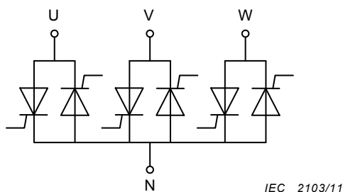
Figure 16 – Montage triphasé en étoile avec neutre
