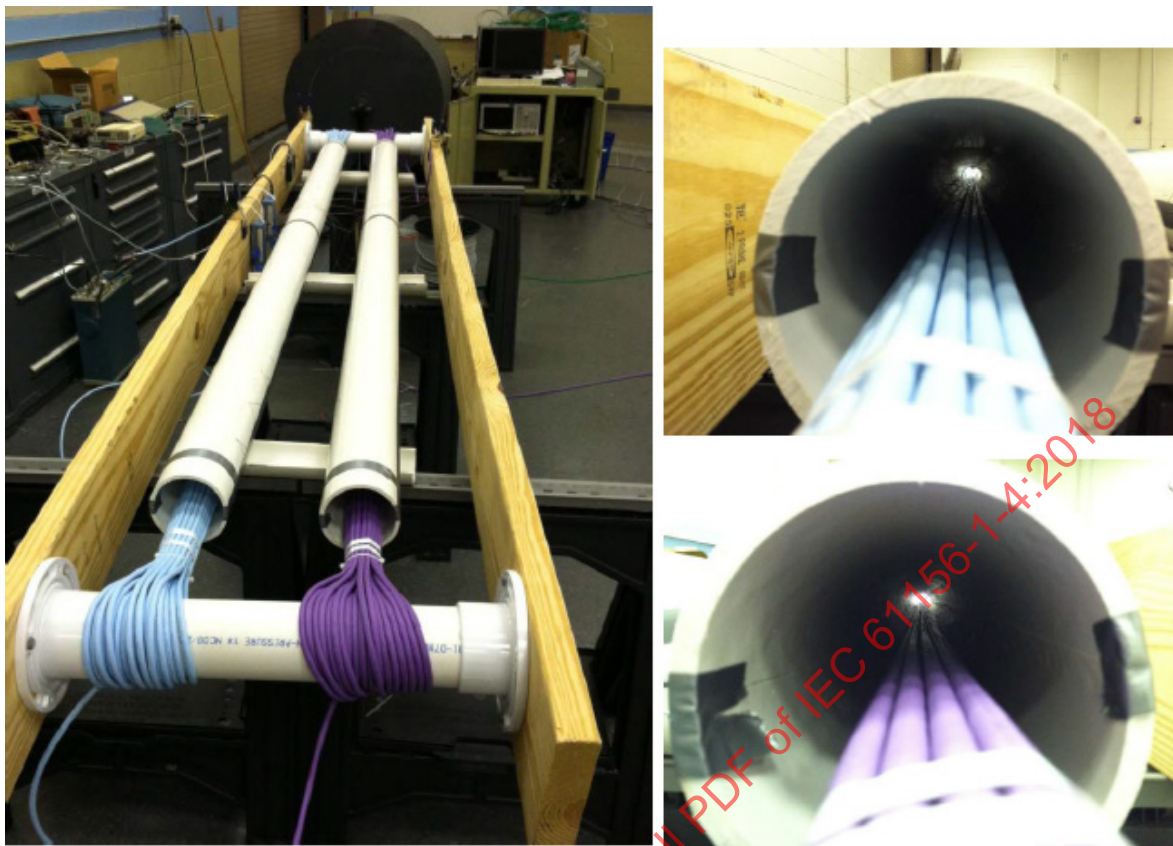
Figure 5 – Conduit
