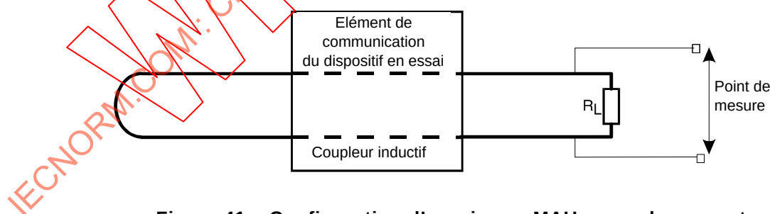
Figure 41 – Configuration d'essai pour MAU en mode courant
