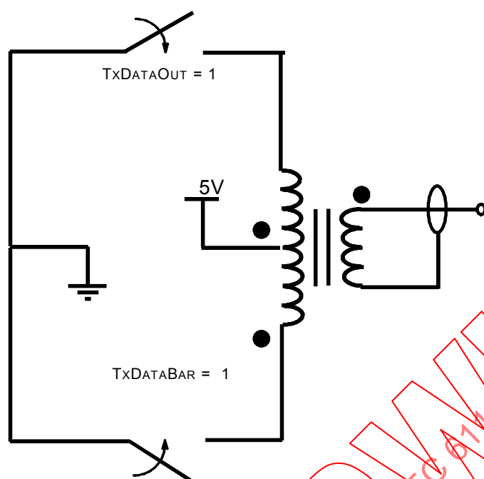
Figure 79 – Emetteur-récepteur de MAU à câble coaxial
