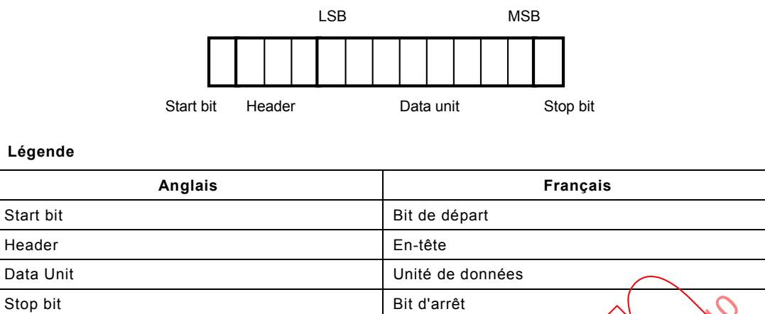
Figure 36 – PhPDU de séquence de données
