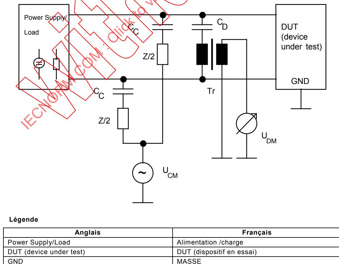
Figure 94 – Schéma de principe de mesure du CMRR
