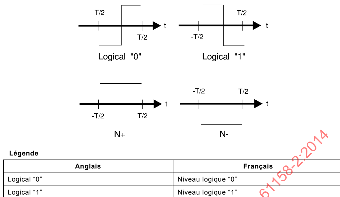
Figure 51 – Règles de codage Manchester
