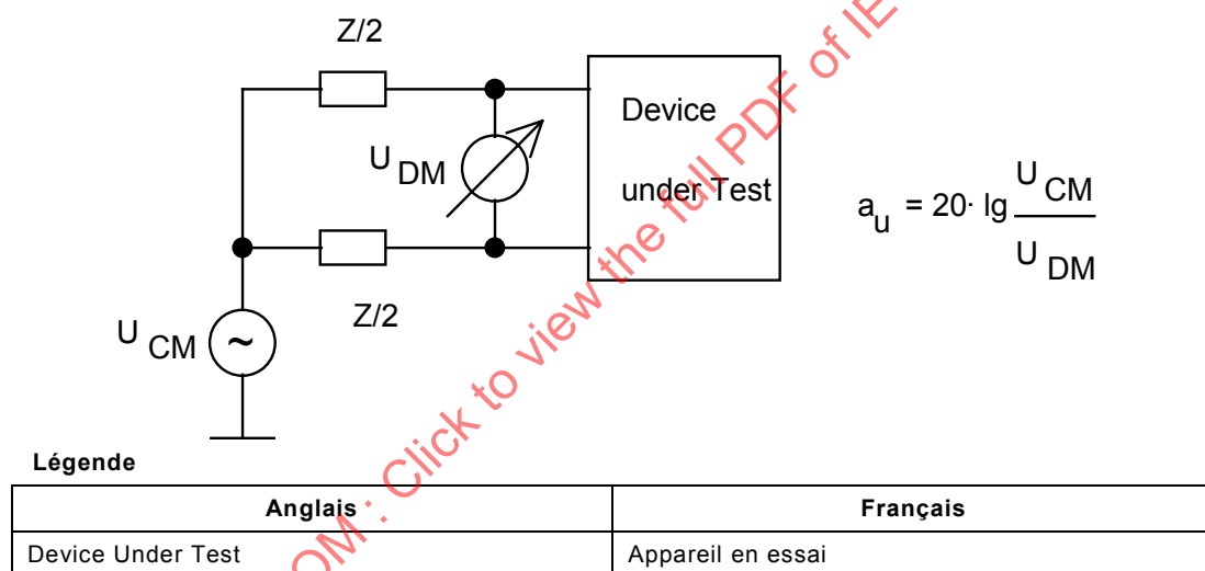
Figure 92 – Définition du CMRR
