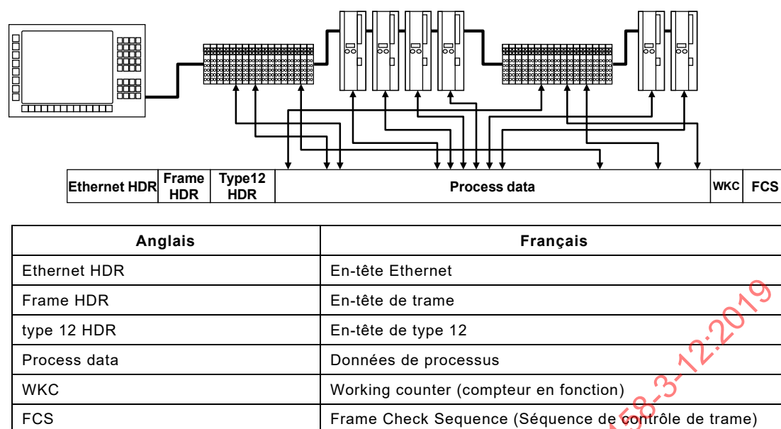
Figure 1 – Mapping des données logiques dans une trame Ethernet composée d'une seule DLPDU de type 12
