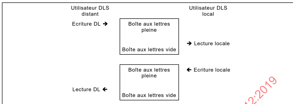
Figure 32 – Interaction de boîte aux lettres SyncM
