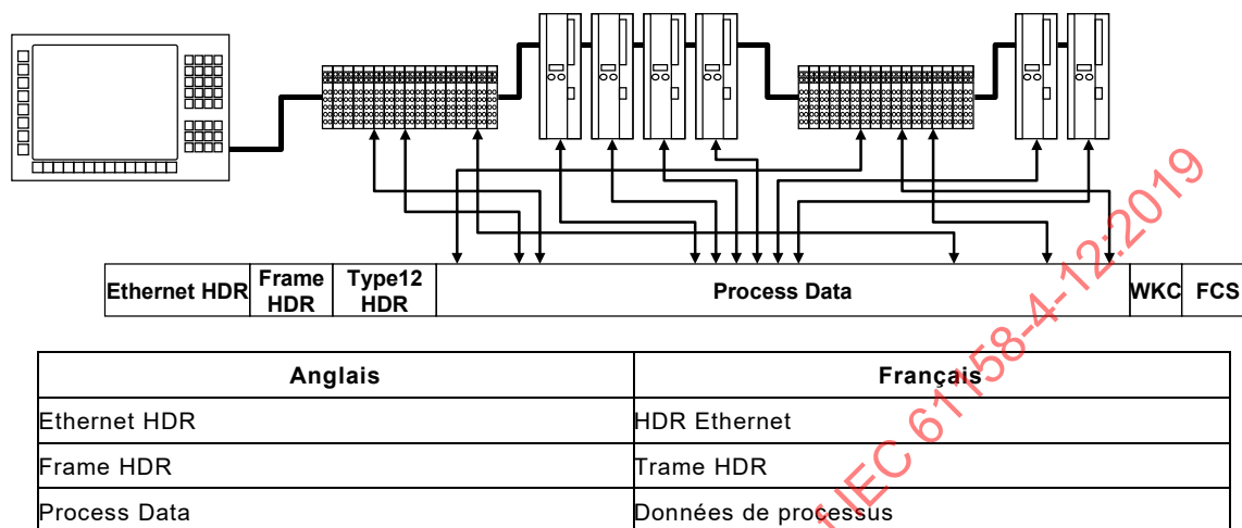
Figure 4 – Mapping des données dans une trame
