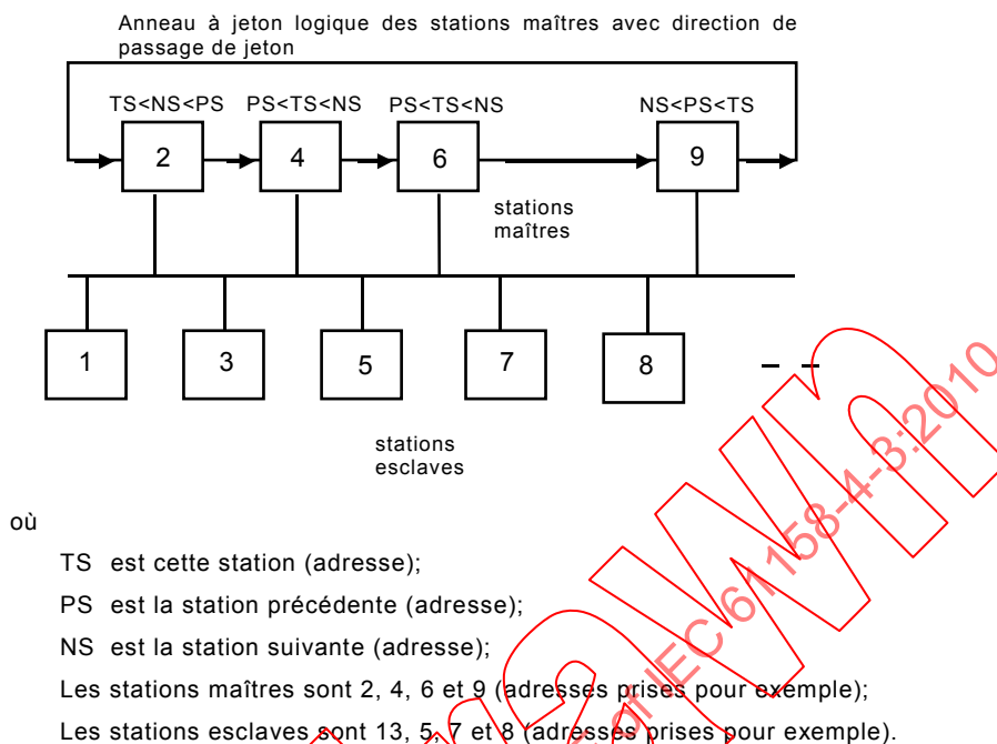
Figure 2 – Anneau logique de passage de jeton
