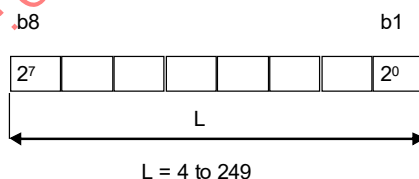
Figure 15 – Codage d'octet de longueur
