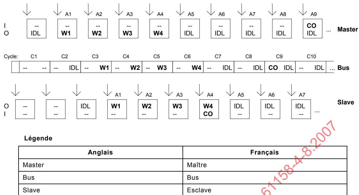
Figure 23 – Transmission de message: maître → esclave
