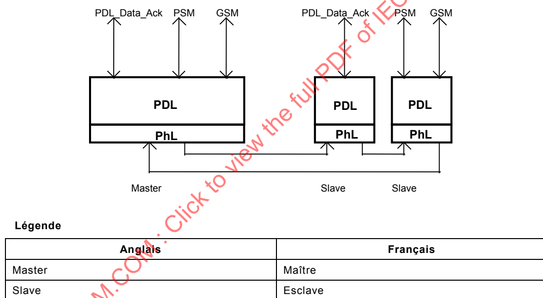
Figure 8 – Vue d'ensemble des services de la PDL
