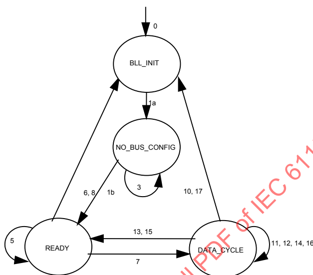
Figure 47 – Machine de protocole de fonctionnement de la BLL du maître
