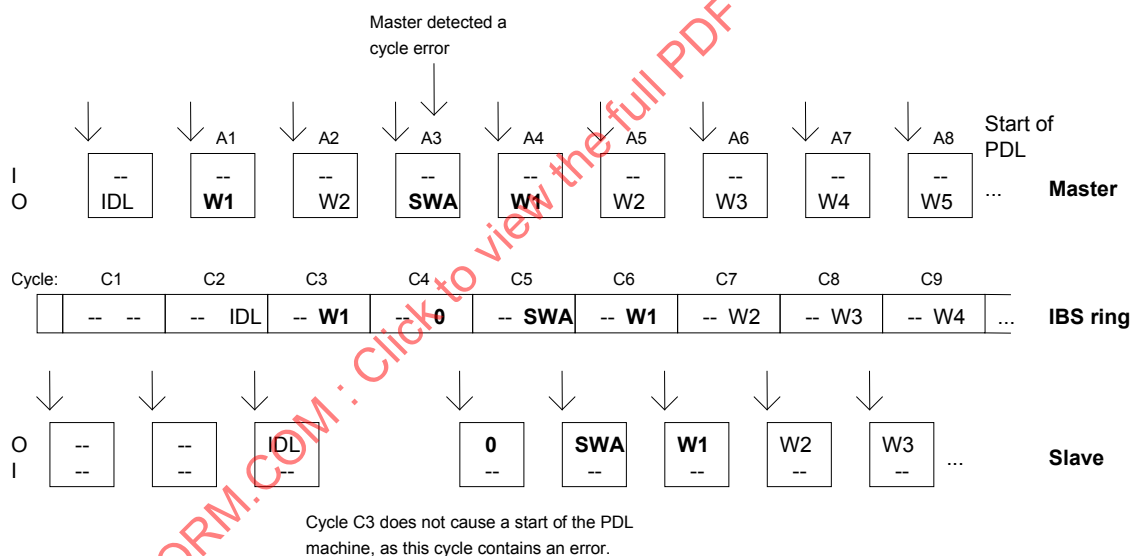
Figure 18 – Transmission de données maître → esclave avec Message SWA
