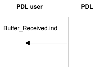
Figure 12 – Service Buffer_Received pour indiquer un transfert de données réussi
