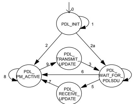
Figure 36 – Machine de protocole de base de la PDL
