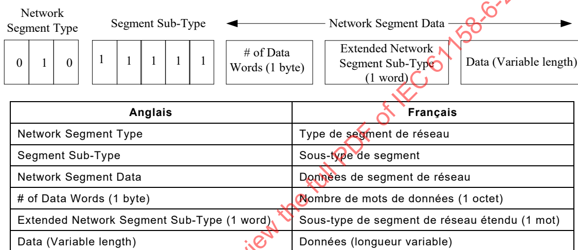
Figure 12 – Segment de réseau étendu
