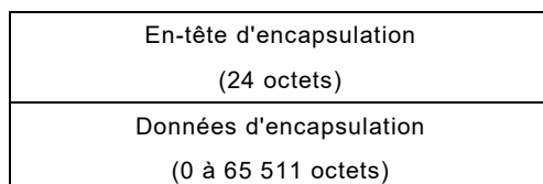
Figure 14 – Message d'encapsulation
