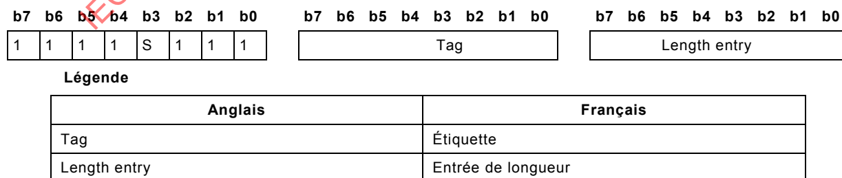
Figure 13 – ID-info pour tag 15 .. 255, length entry 7 .. 255
