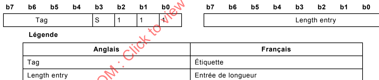
Figure 12 – ID-info pour tag 0 .. 14, length entry 7 .. 255
