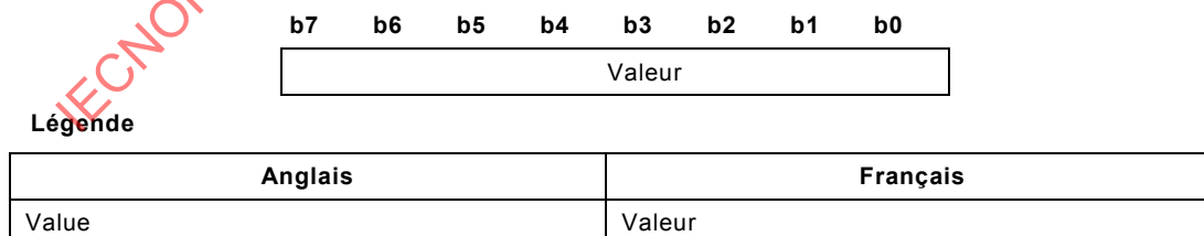
Figure 7 – Codage d'une valeur marquée PRIVATE
