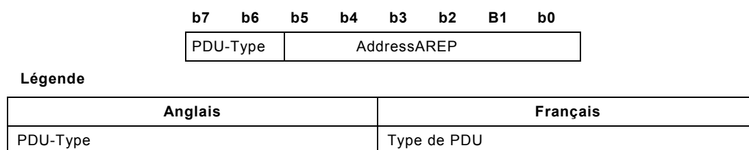
Figure 2 – En-tête d'APDU
