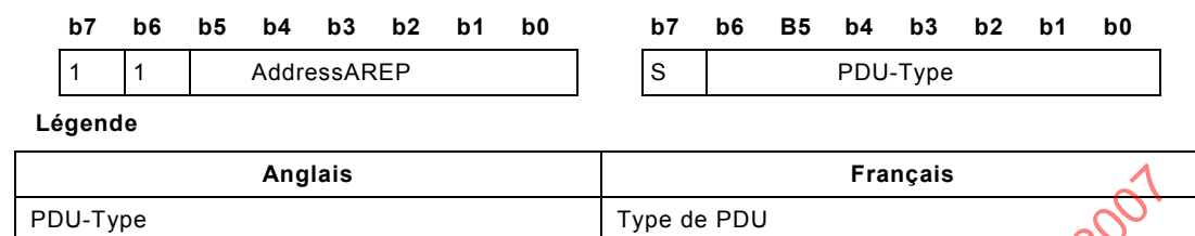
Figure 3 – PDU avec extension de type
