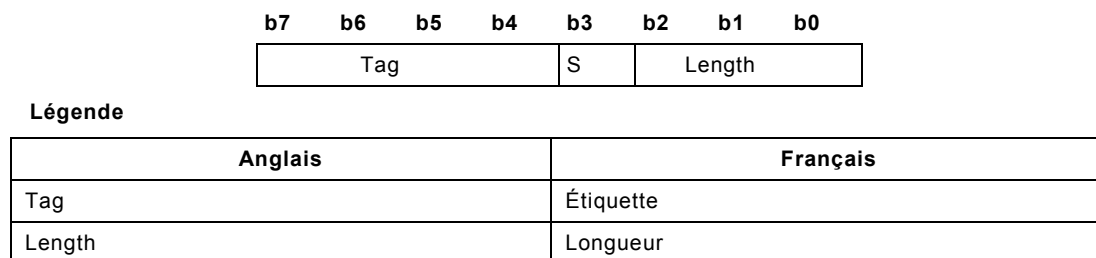
Figure 10 – ID-info pour tag 0 .. 14, length entry 0 .. 6
