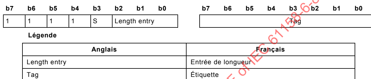
Figure 11 – ID-info pour tag 15 .. 255, length entry 0 .. 6
