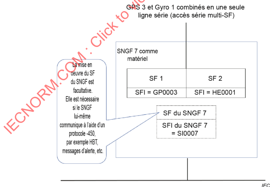
Figure 3 – Exemple de SNGF, accès série multi-SF
