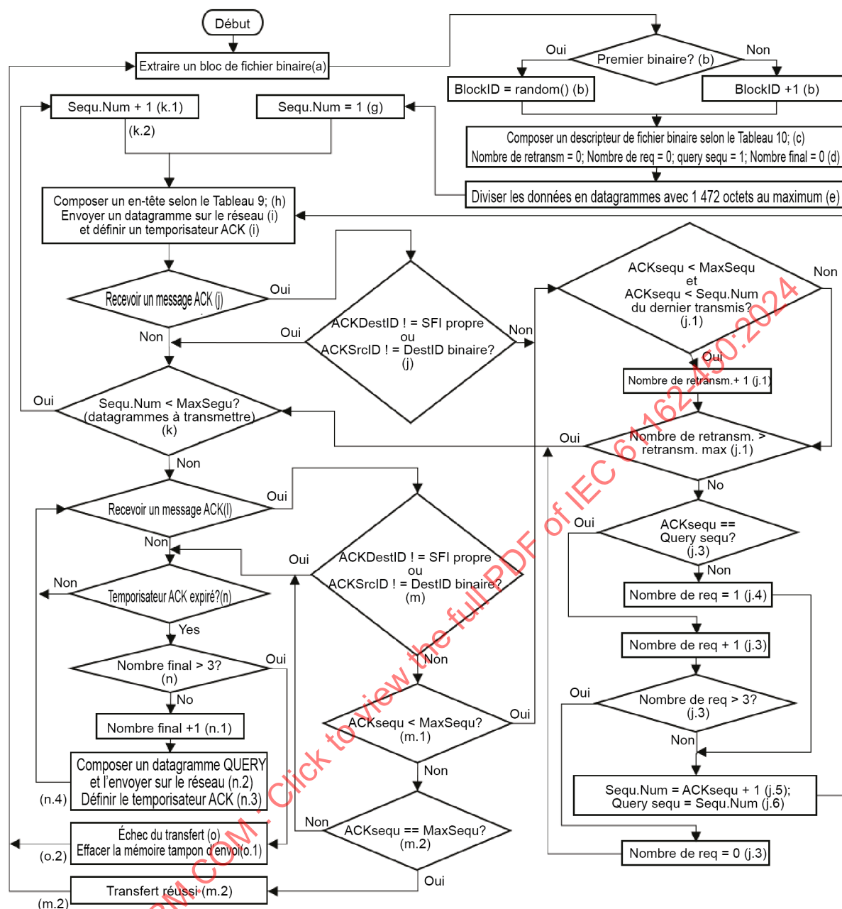
Figure 6 – Processus d'envoi retransmissible
