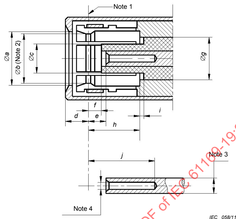
Figure 1 – Connecteur avec contact central femelle (pour les dimensions et les notes, voir le Tableau 1)
