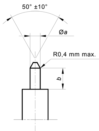
Figure 3 – Broches calibrées pour contact central femelle (pour les dimensions, voir le Tableau 3)
