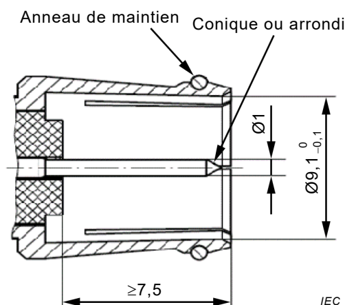
Figure 4 – Exemple de fiche mâle de connecteur de type "F-Quick" avec conducteur extérieur fendu et un anneau de maintien (usage intérieur)
