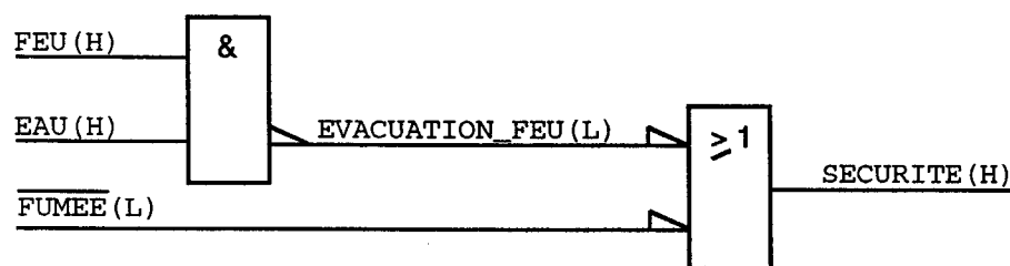
Figure 11 - Indications de polarité et niveaux de signal
