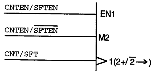
Figure 9 - Exemple de dénominations de signaux pour signaux à fonctions multiples
