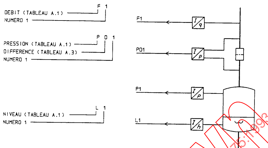
Figure 7 - Exemple de dénominations de signaux codés pour signaux analogiques - circuit mesurant les grandeurs non électriques
