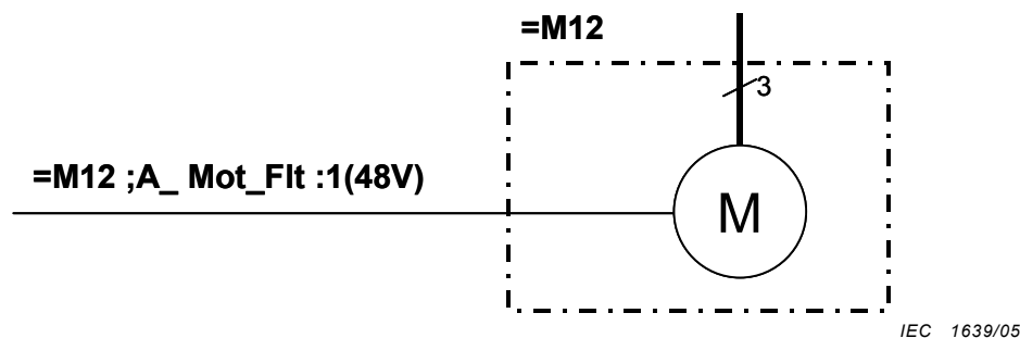
Figure 21 – Exemple de désignation d'un signal correspondant à la classe de conformité 2
