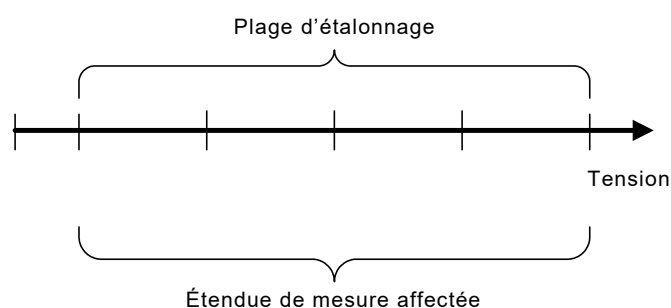
Figure 2 – Étalonnage par comparaison sur la plage de pleine tension
