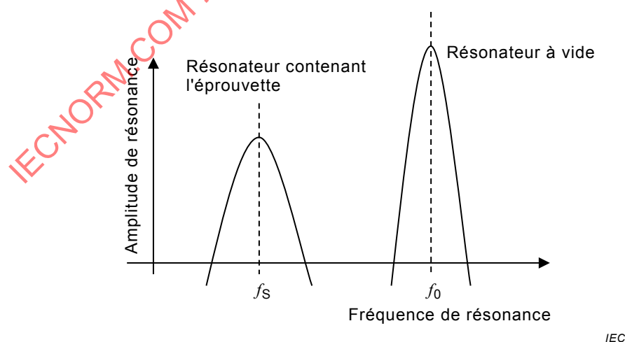
Figure 3 – Schéma montrant le changement de fréquence de résonance avec ou sans éprouvette
