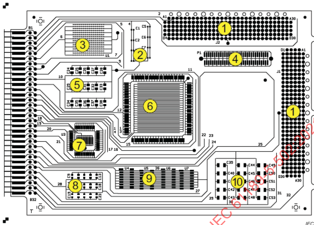
Figure 2 – IPC-B-52 Rev B en vue de dessus
