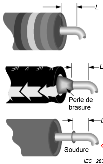
Figure 1 – Formation des sorties, extension des sorties
