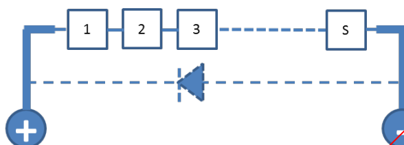
Figure 1 – Cas S, connexion série avec diode de dérivation facultative
