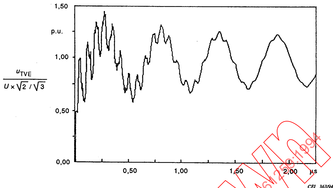
Figure 2 – Forme typique de tension (comportant les composantes VFT et FT)
