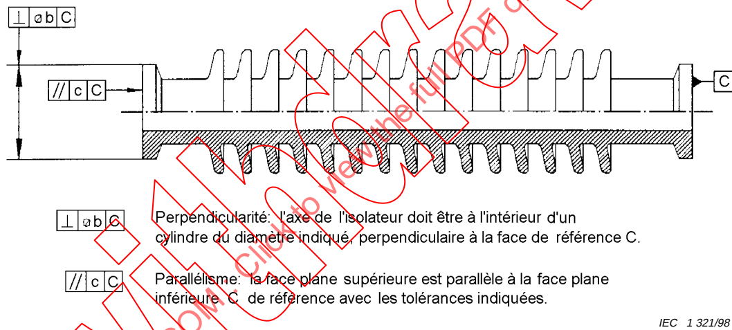
Figure A.5 – Parallélisme et perpendicularité
