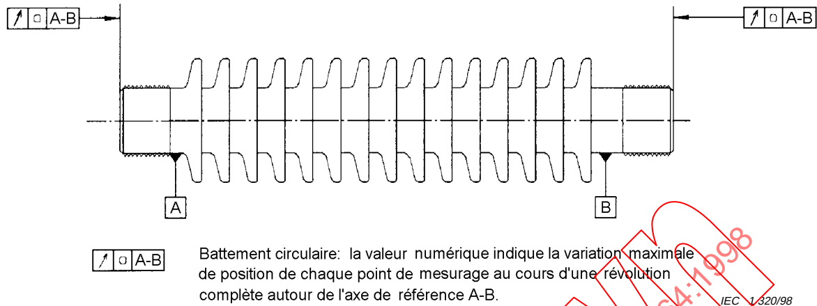
Figure A.4 – Battement circulaire
