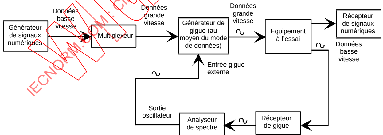
Figure 3 – Configuration pour la mesure de la fonction transfert de gigue – technique par démultiplexage
