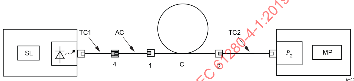
Figure C.2 – Mesure d'essai
