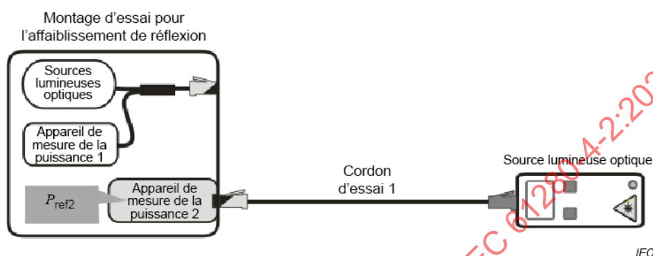
Figure F.2 – Mesurage de l'affaiblissement interne du système P_{ref2}
