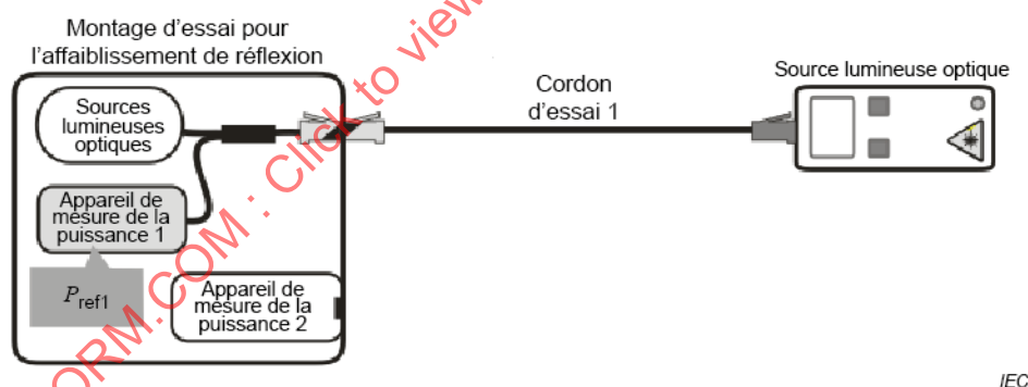
Figure F.3 – Mesurage de l'affaiblissement interne du système P_{ref1}
