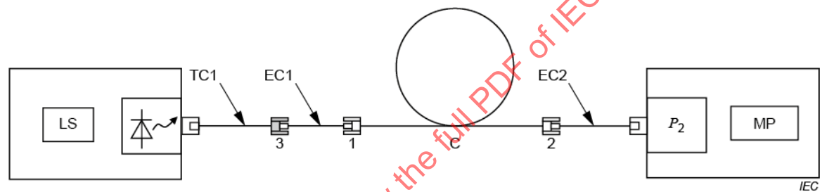
Figure D.1 – Mesure de référence
