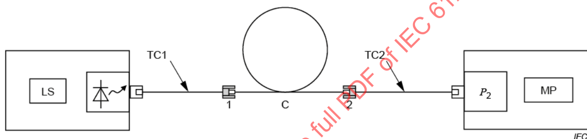
Figure B.1 – Mesure de référence à trois cordons
