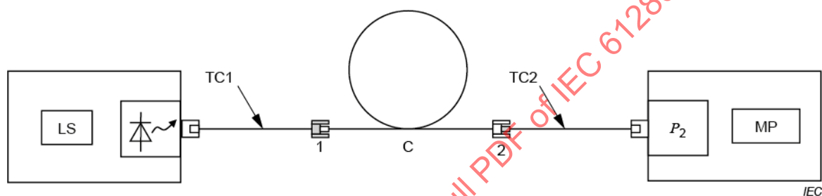
Figure C.1 – Mesure de référence à deux cordons
