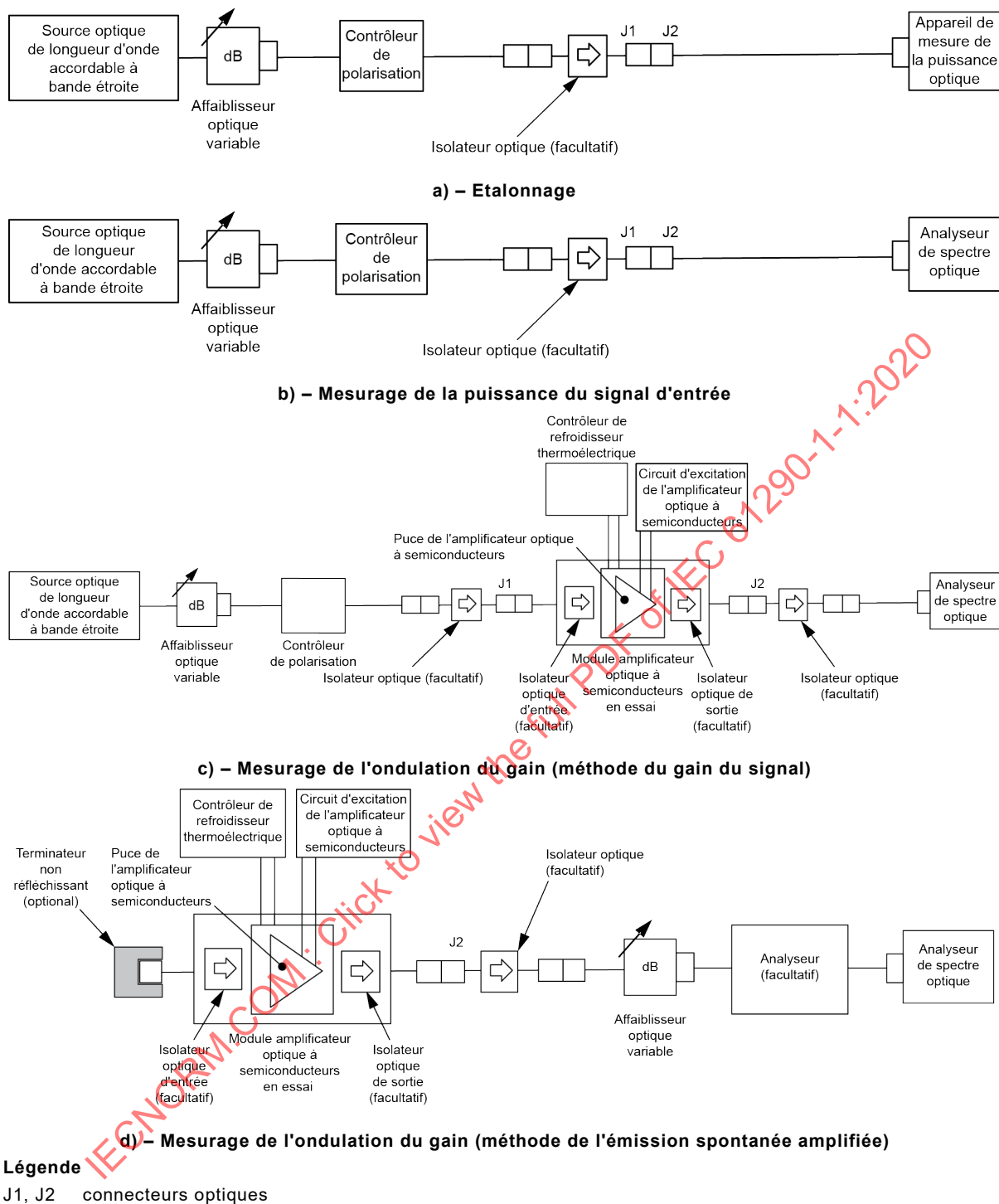
Figure 2 – Organisation typique de l'appareillage d'essai de l'analyseur de spectre optique pour les mesurages de l'ondulation du gain
