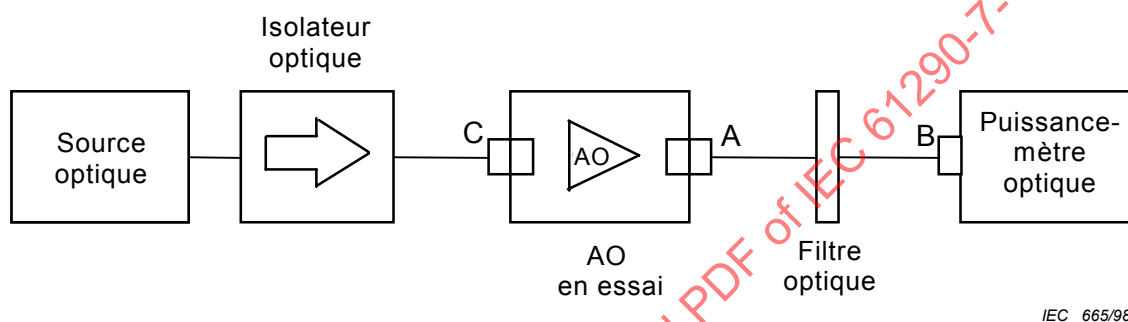
Figure 1b – Mesure de la perte d'insertion hors-bande
