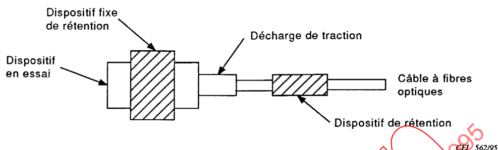
Figure 1 - Montage d'essai
