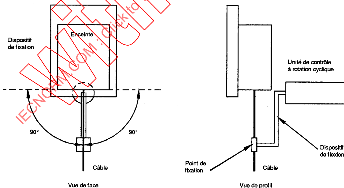
Figure 1 – Appareillage d'essai
