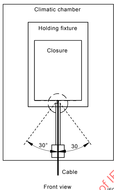
Figure 1 – Appareillage d'essai
