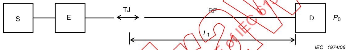
Figure 2a – Affaiblisseurs non connectés avec fibres amorce fixées
