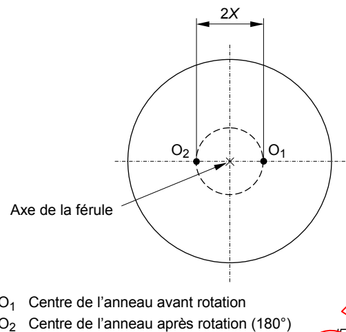
Figure 2a – Mesure idéale, quand le système de mesure n'introduit pas de désalignement
