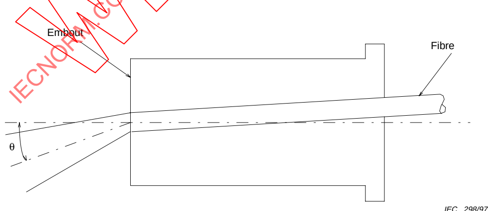
Figure 1 – Définition de l'erreur d'alignement angulaire
