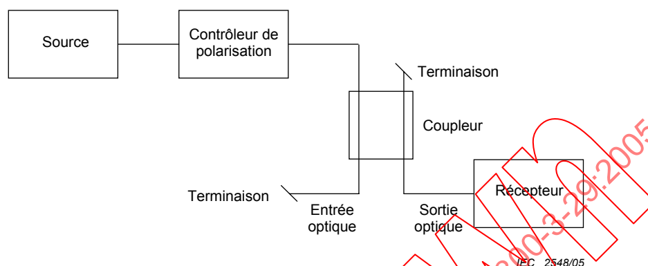
Figure A.3 – Montage pour la mesure de la constante du système
