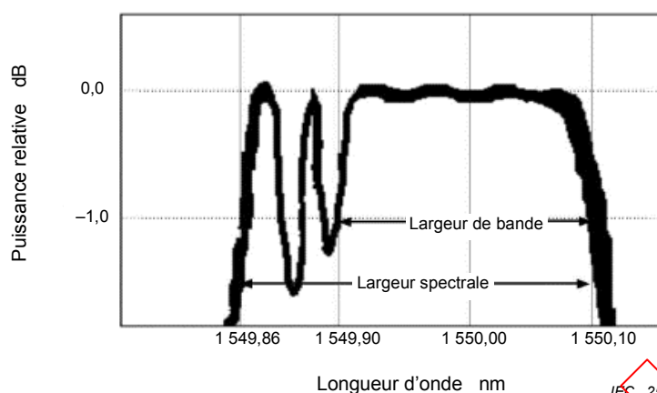
Figure 6 – Largeur de bande et largeur spectrale totale pour un réseau de Bragg sur fibre
