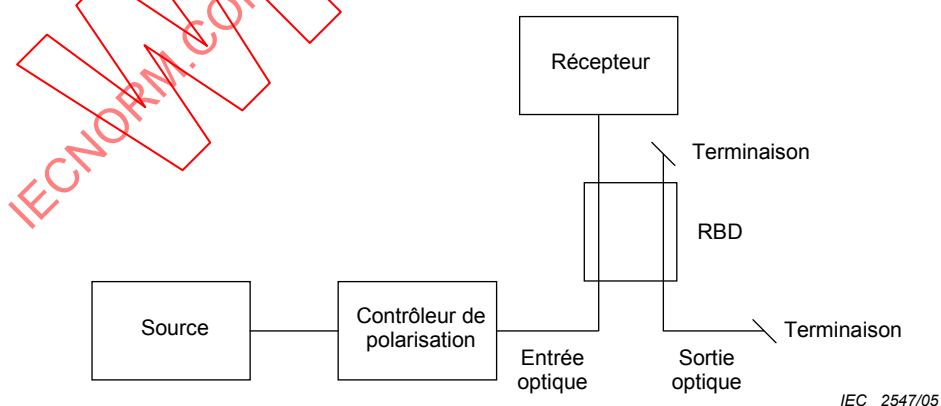
Figure A.2 – Montage de référence de la source
