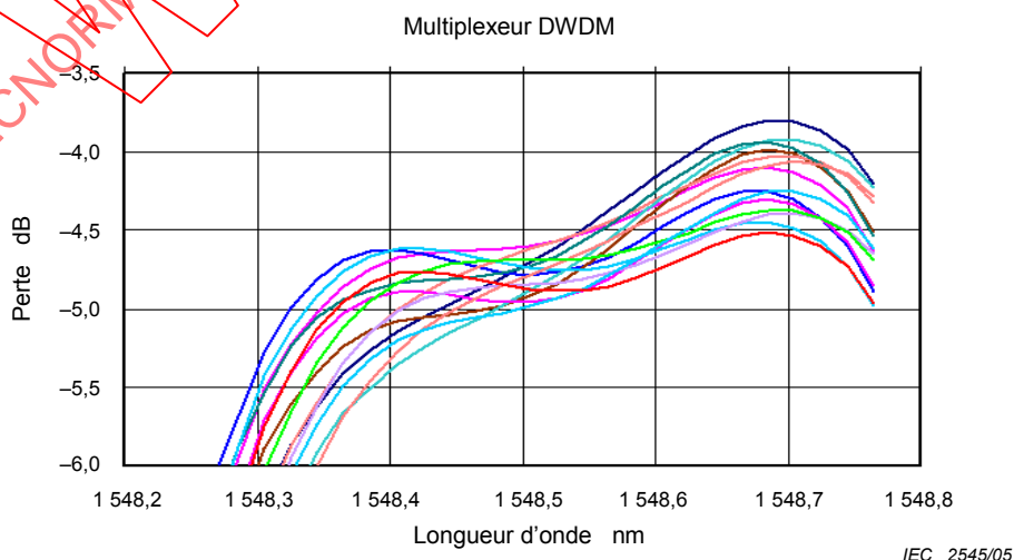
Figure 8 – Dépendance à la polarisation de la fonction de transfert
