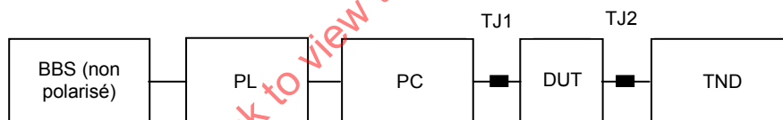
Figure 3 – Montage de mesure pour système avec TNLS et détecteur ajustable à bande étroite (TND)
