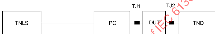
Figure 2 – Montage de mesure pour système avec source de rayonnement lumineux ajustable à bande étroite (TNLS)
