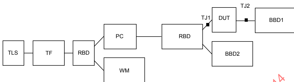
Figure 2 – Montage de mesure pour système avec source de rayonnement lumineux ajustable à bande étroite (TNLS)
