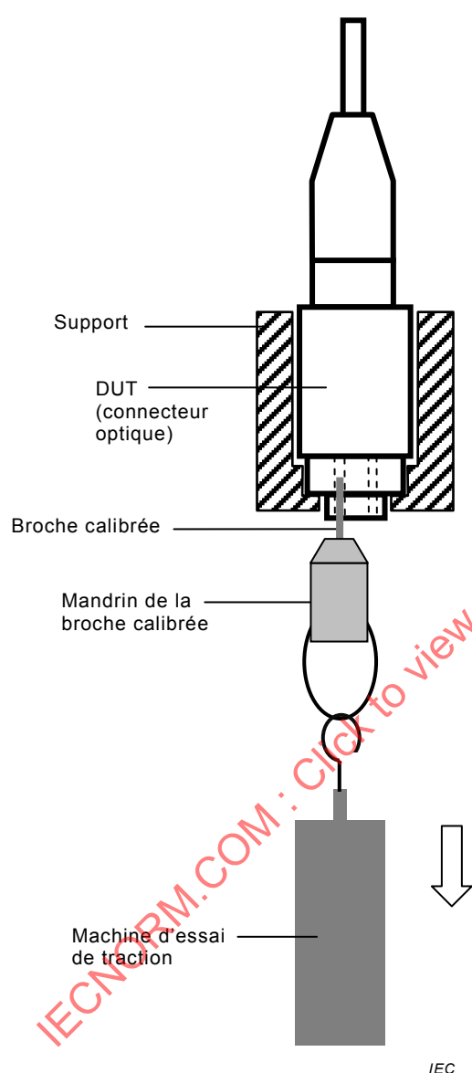
Figure 4a – Mesure pour alésage unique
