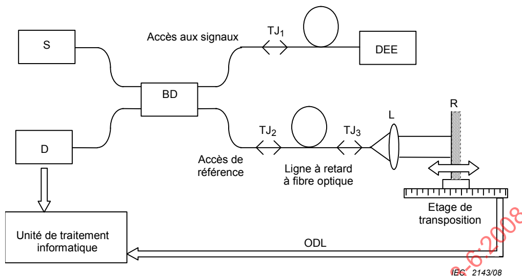
Figure 3 – Montage de mesure de l'affaiblissement de réflexion par la méthode OLCR
