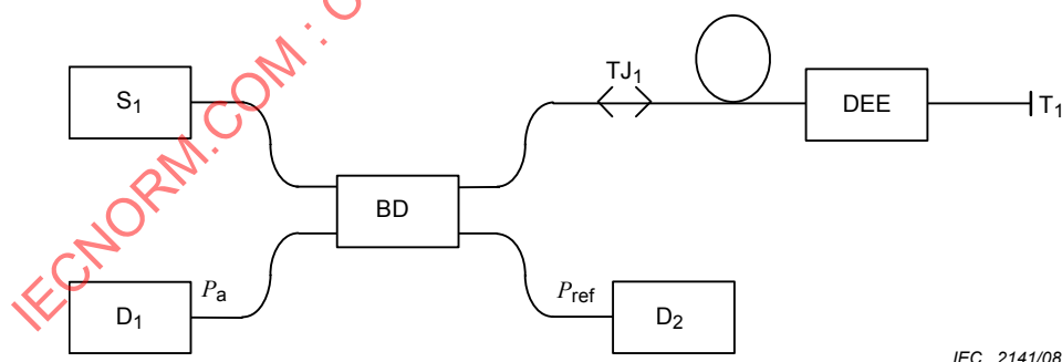
Figure 1 – Montage de mesure de l'affaiblissement de réflexion par la méthode OCWR
