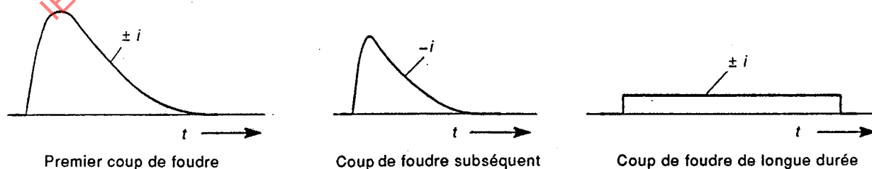
Figure 1 – Définitions des paramètres des coups de foudre
