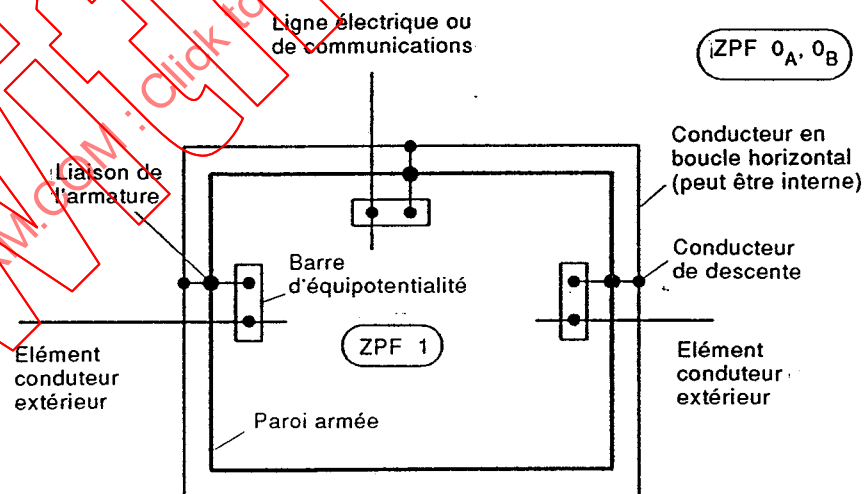
Figure 11 – Liaison d'équipotentialité dans le cas de points d'entrée multiples au niveau du sol d'éléments conducteurs extérieurs
