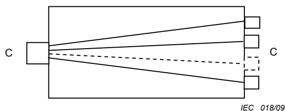
Figure 2 – Système d'éclatement semi-compact
