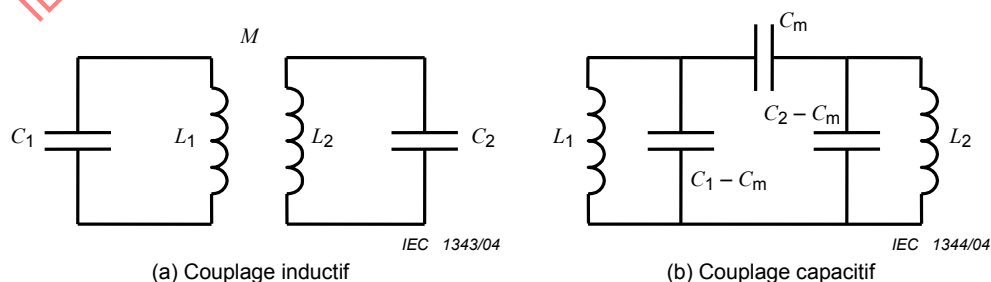
Figure 1 – Circuit équivalent
