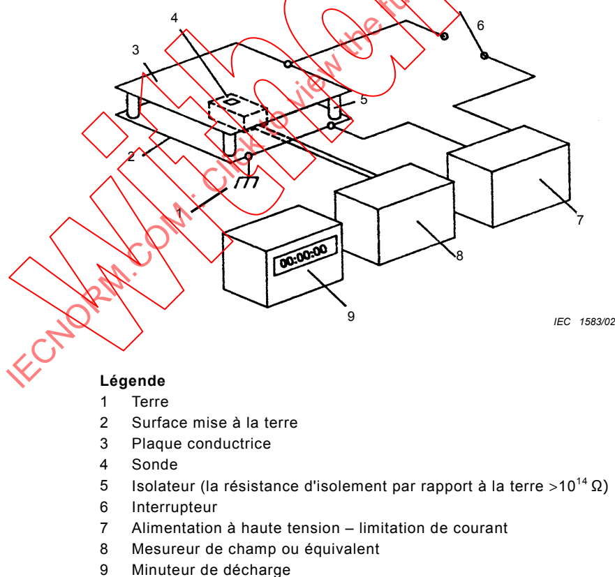
Figure 2 – Composants de moniteur à plaque chargée 2
